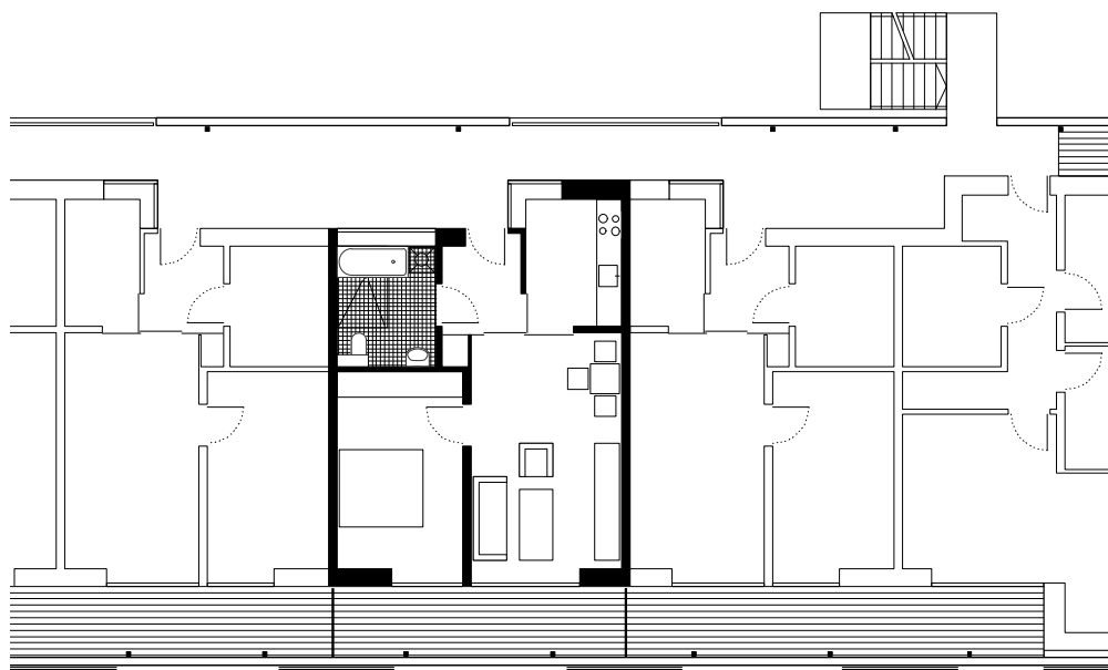
54 Grundriss Whg. M 1:200
