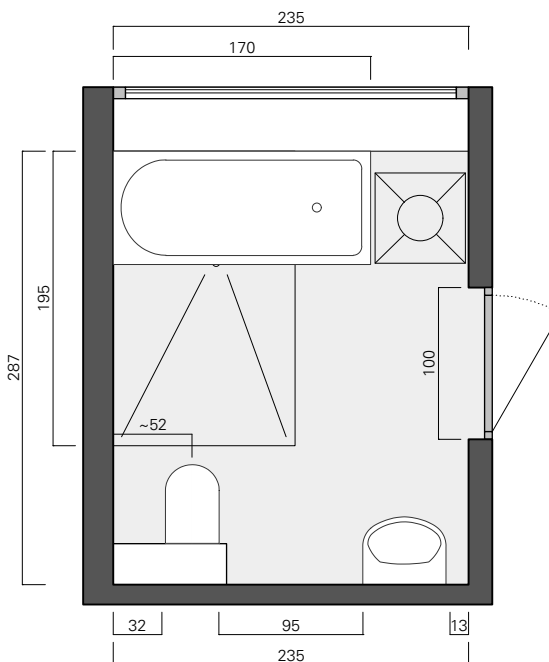
55 Grundriss Bad M 1:50
