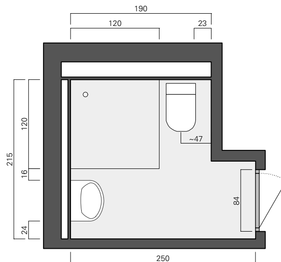
67 Grundriss Bad M 1:50
