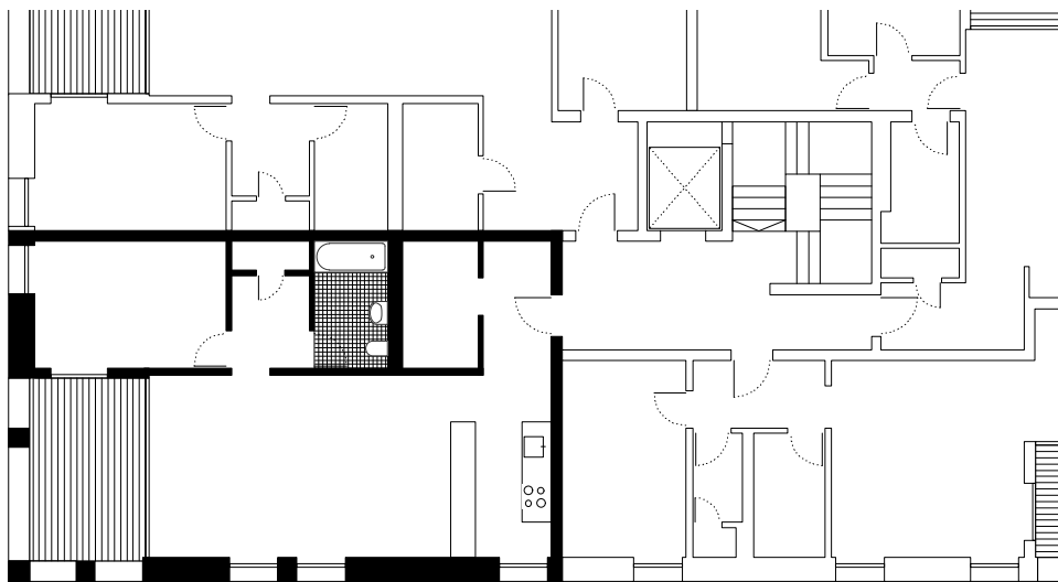
73 Grundriss Whg. M 1:200
