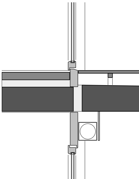
62 Detail Balkon M 1:20
