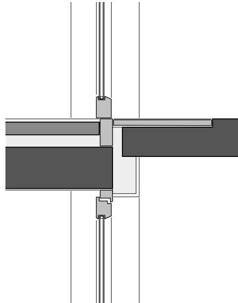
63 Detail Wohnungstür M 1:20
