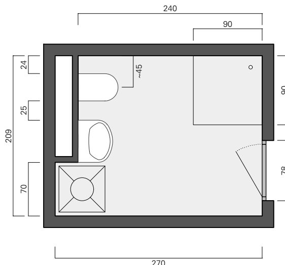
Grundriss (Dusch-)Bad M 1:50
