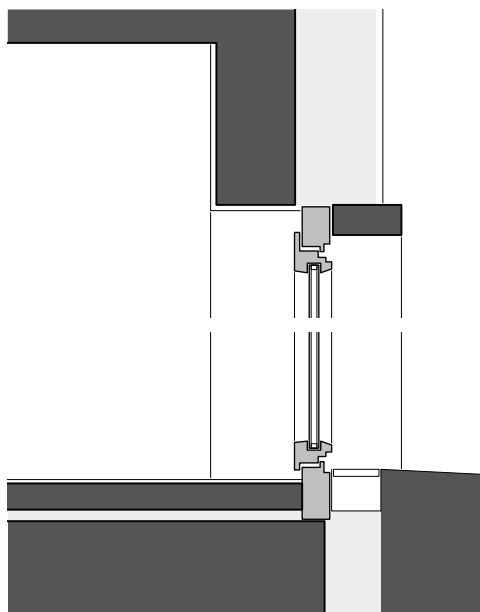
68 Detail Terrasse M 1:20
