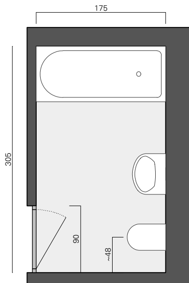
74 Grundriss Bad M 1:50
