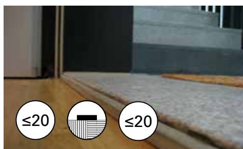
Wohnungseingang (Perspektive)
