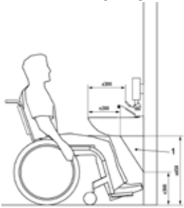
Ansicht (Seite) M 1:100 Quelle: ISO 21542:2011, Bild 44
