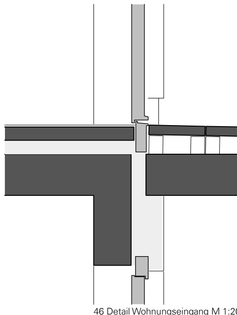
46 Detail Wohnungseingang M 1:20
