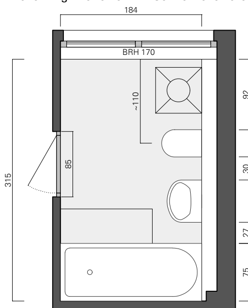
61 Grundriss Bad M 1:50
