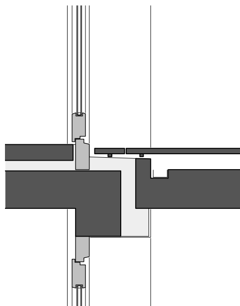
50 Detail Balkon M 1:20
