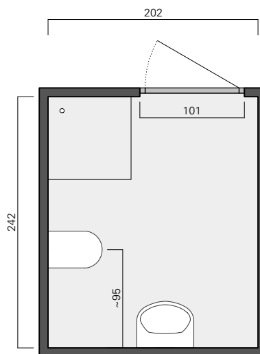
88 Grundriss Bad M 1:50
