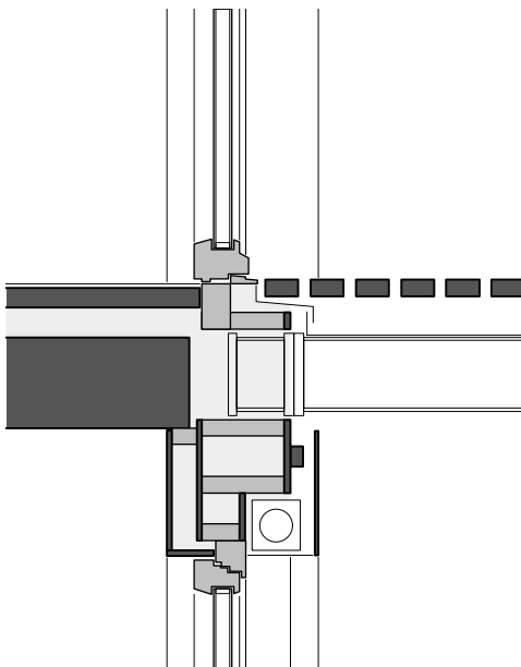
39 Detail Balkenschwelle M 1:20
