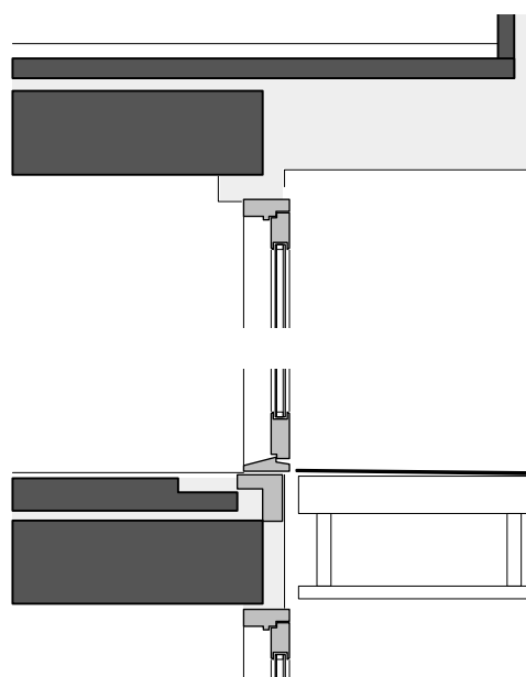
90 Detail Balkontür M 1:20
