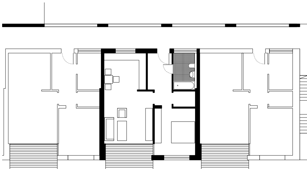
60 Grundriss Whg. M 1:200
