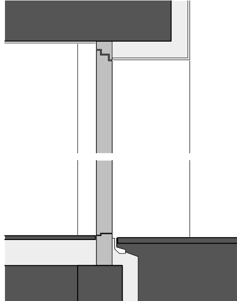
51 Detail Hauseingang M 1:20
