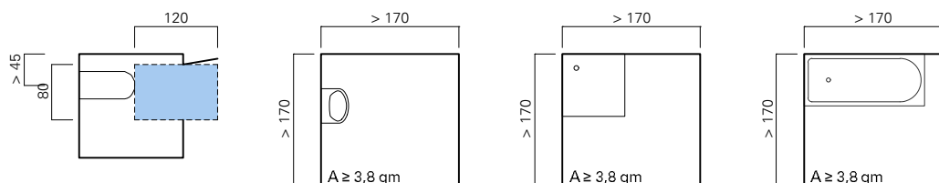
Abb. 5 Anpassbarer Bad-/Duschraum nach SIA 500:2009, 10.2.1 Schweizer Anforderungen an Nutz- und Bewegungsflächen für das hindernisfreie WC bzw. Bad
