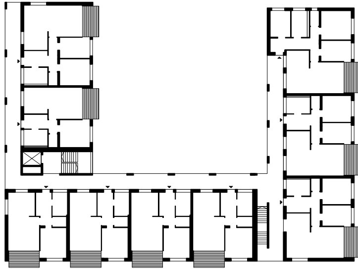
59 Grundriss RG M 1:500
