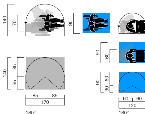
Grundrisse M 1:100 Abb. 9 ready Bewegungsfläche
