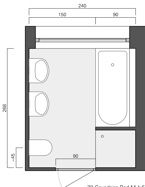
78 Grundriss Bad M 1:50
