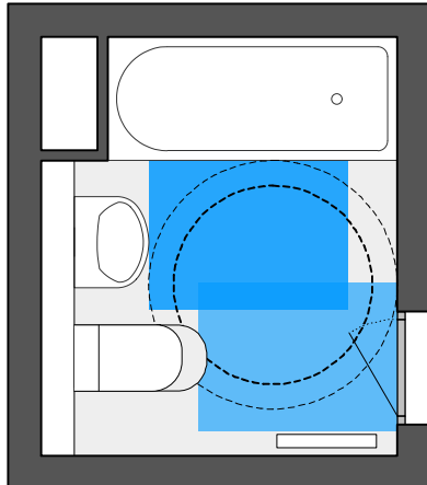
05 170 (190) x 175 (250) = 4,8 m 2
