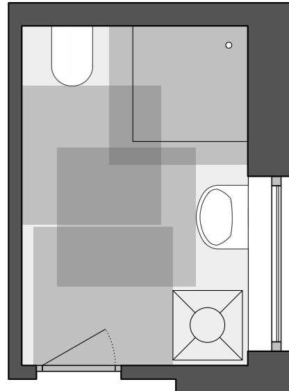
06 1,84* x 3,93* = 7,3 m 2
