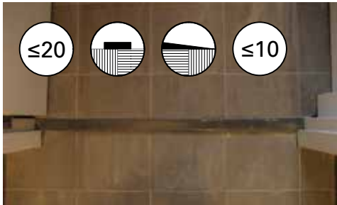
Wohnungseingang (Aufsicht)
