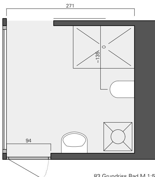
83 Grundriss Bad M 1:50
