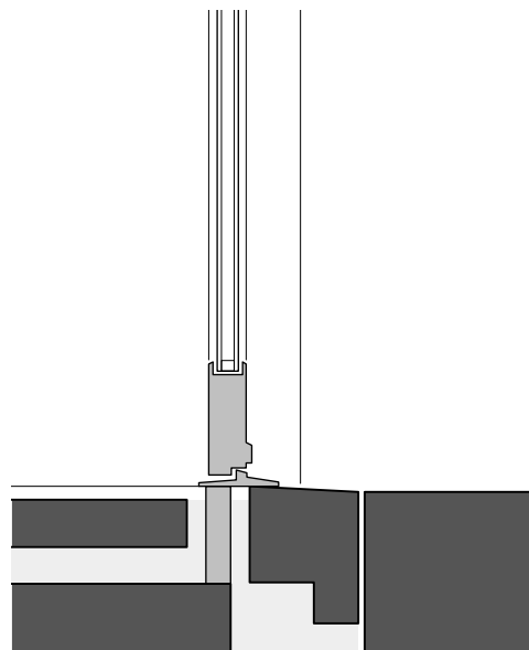
89 Detail Schwelle M 1:10
