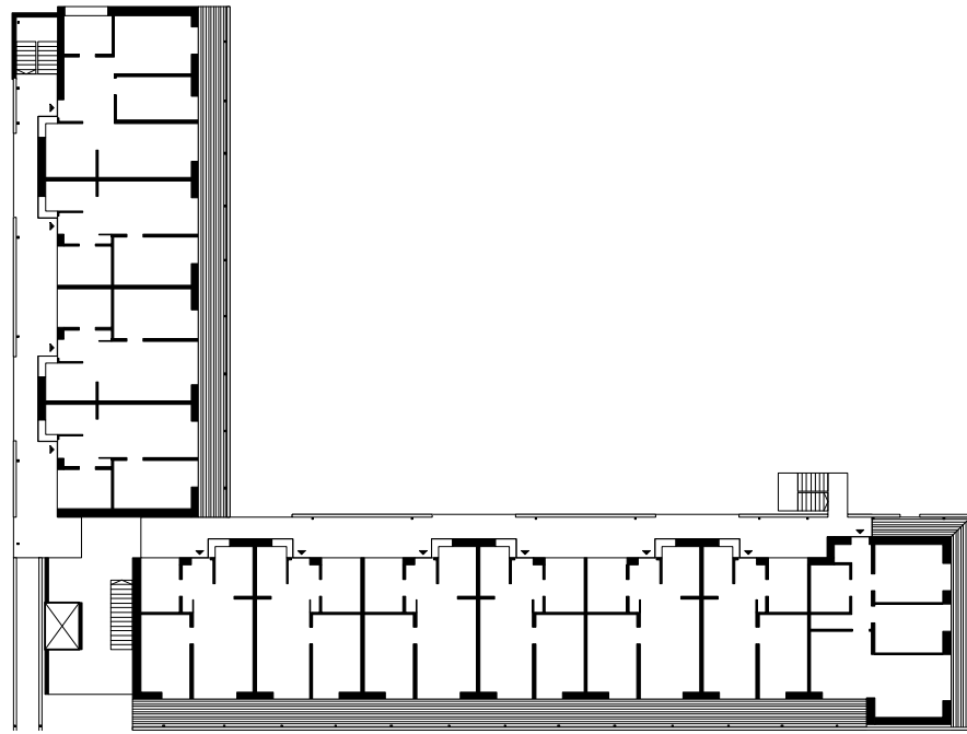
53 Grundriss RG M 1:500
