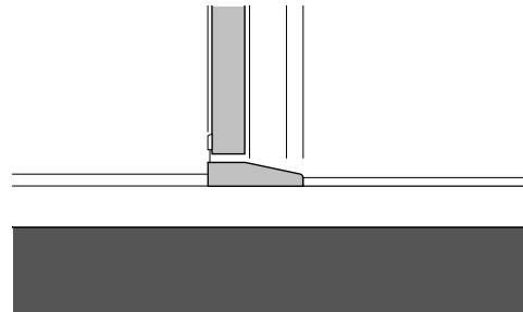
79 Detail Schwelle entsprechend ISO 21542 M 1:10
