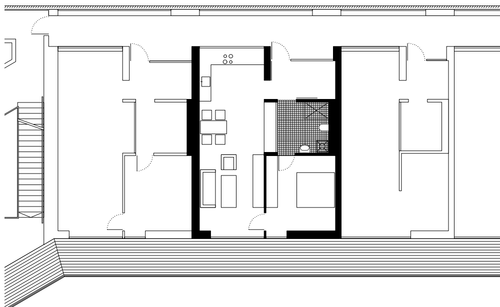
82 Grundriss Whg. M 1:200
