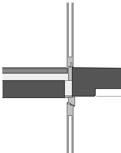
57 Detail Wohnungseingang 1:20
