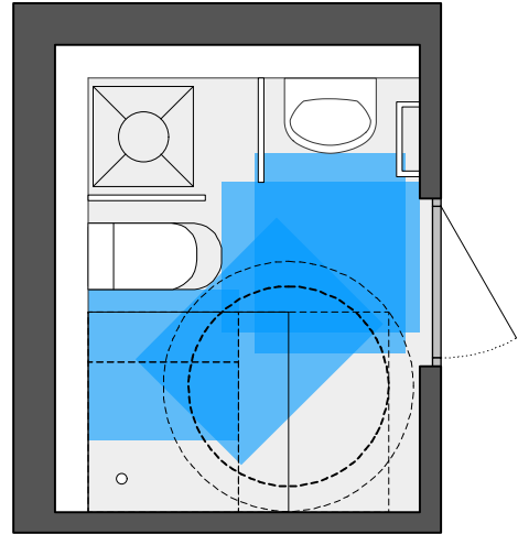
02 200* x 261* = 5,3 m 2
